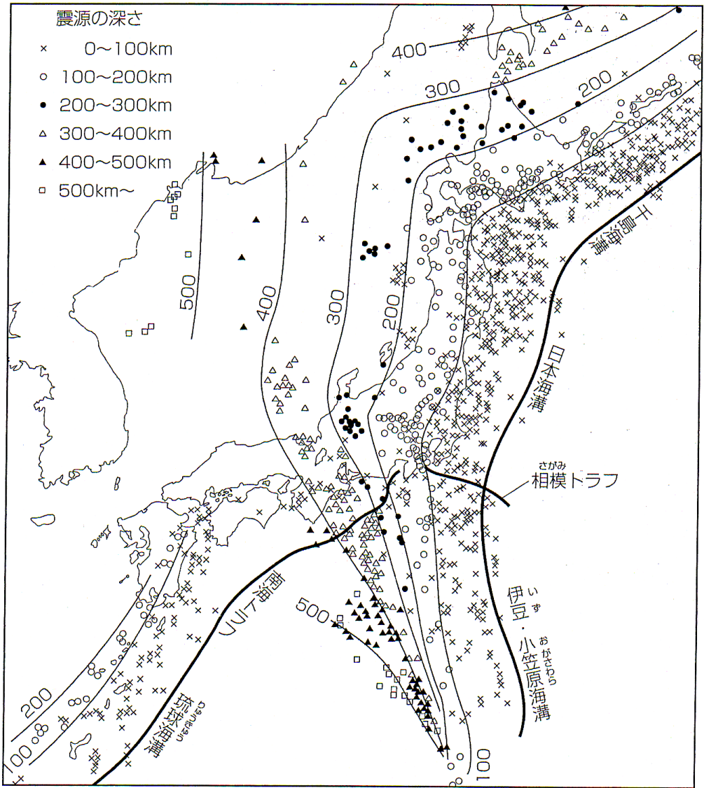
日本列島の地震分布 (吉井敏尅、1978) 21)
